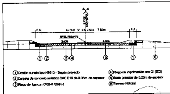
Imagen 05 - Perfil tipo de estructura de pavimento.
