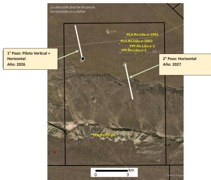
Figura 3. Área Loma Guadaluza: ubicaciones tentativas pozos PLAN PILOTO
